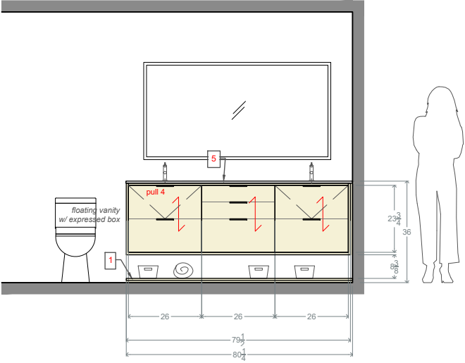
Elevation 1
