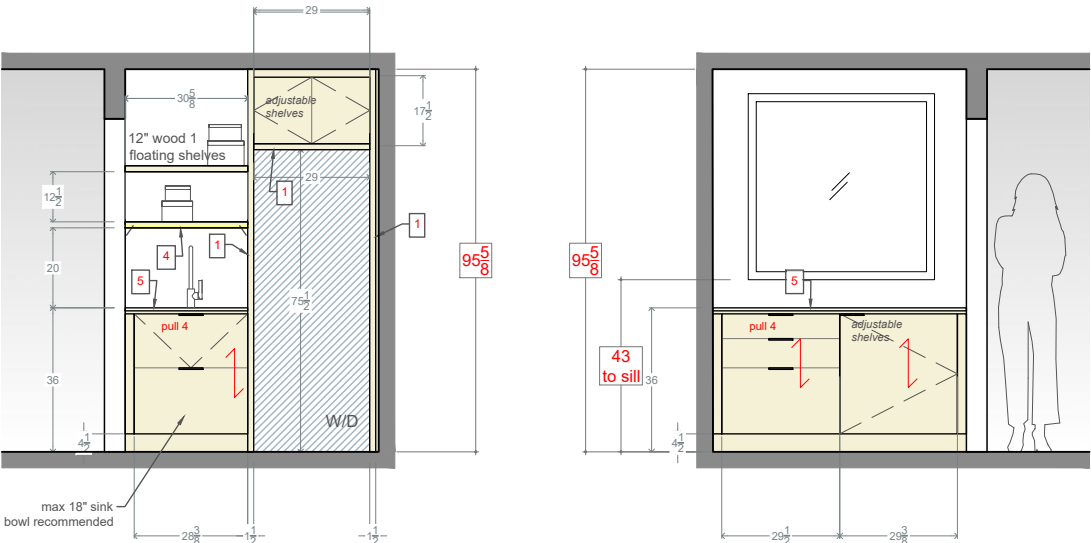
Elevation 1
