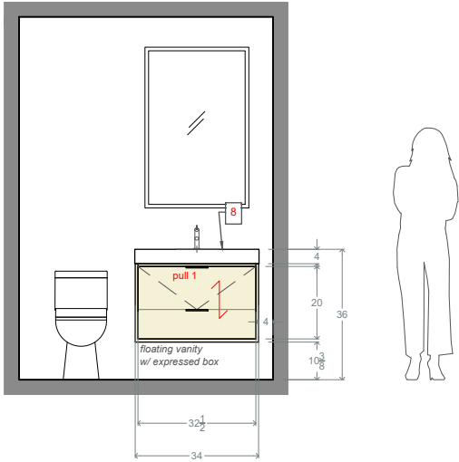
Elevation 1
