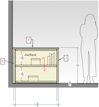
Elevation 3
