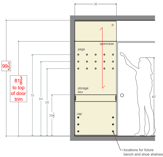
Elevation 1
