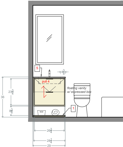
Elevation 1
