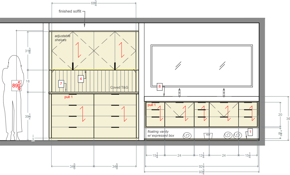
Elevation 1
